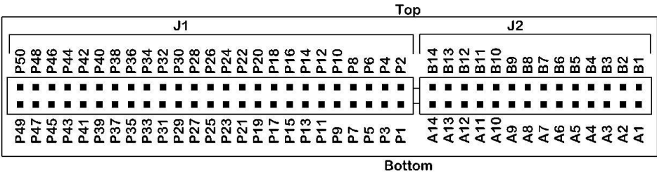
DM5028 模块的 J1、J2 连接件端面引脚分布定义（正视图）
