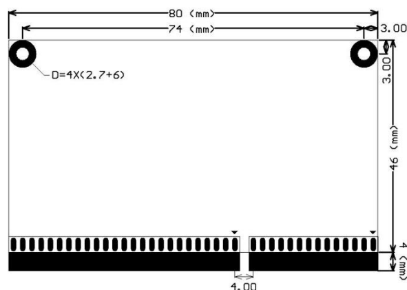
DM5028 标准尺寸
