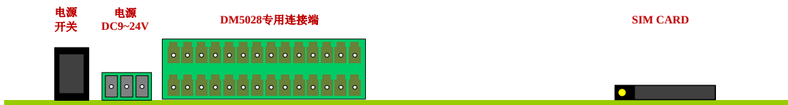
SBC884 端面 2 示意图
