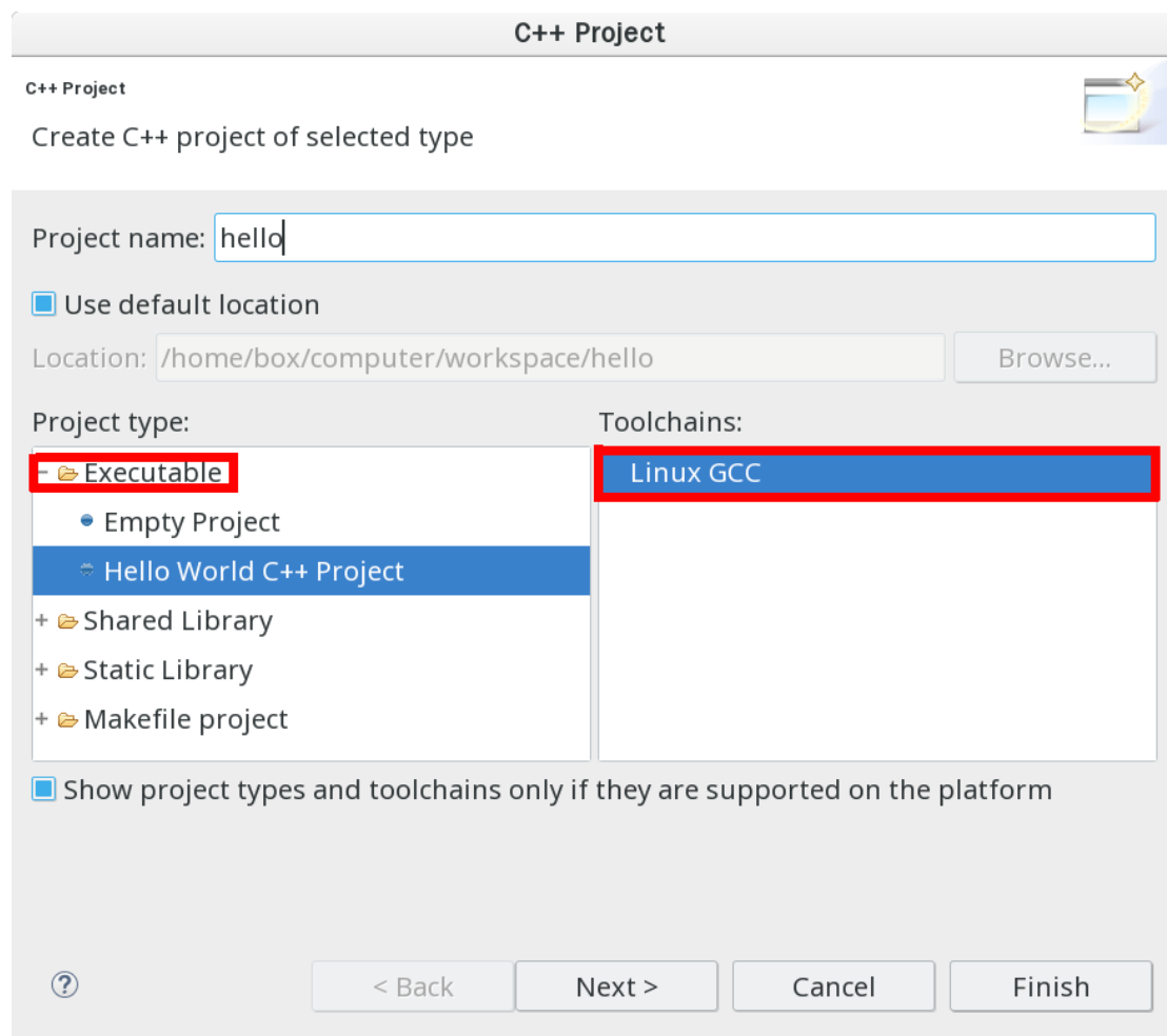
选择 Toolchains
