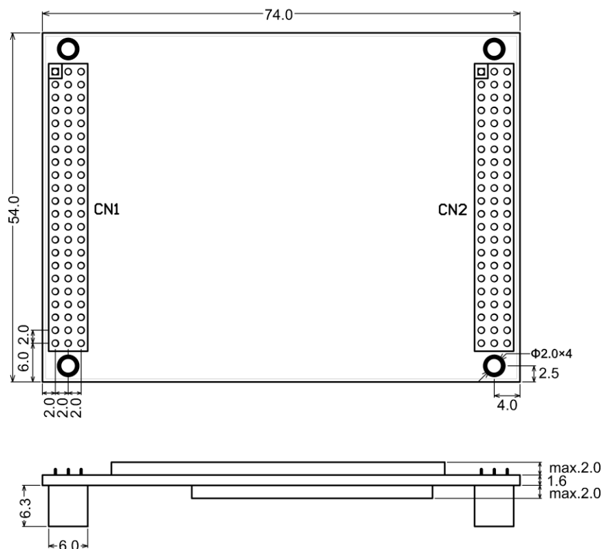
ESM7400 主板外形尺寸示意图（单位：mm）
