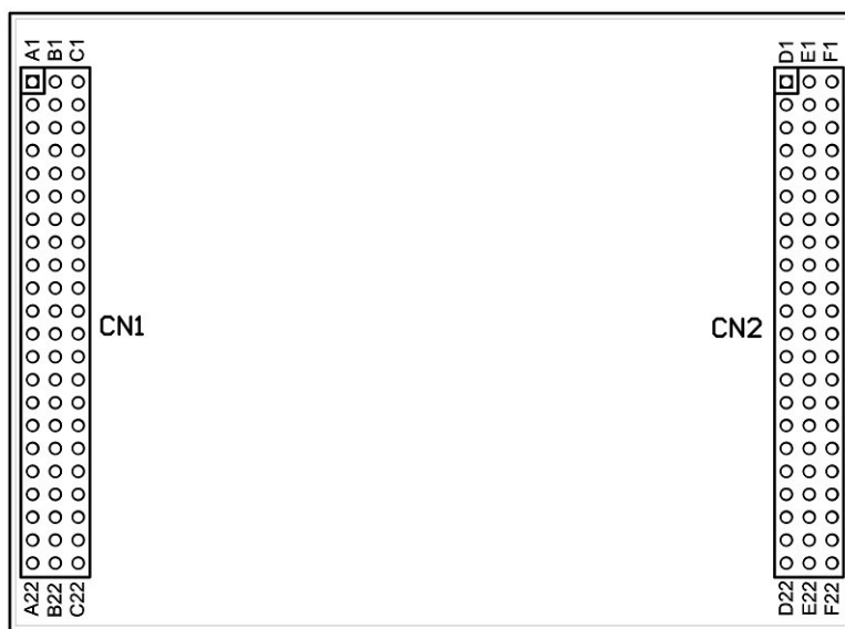
ESM7400 的 CN1、CN2 所在位置示意图
