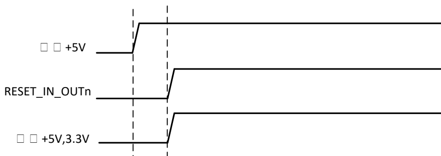
ESM7400 主板上电时时序要求
