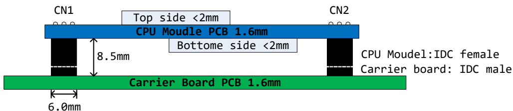
ESM7400 与应用底板结构示意图
