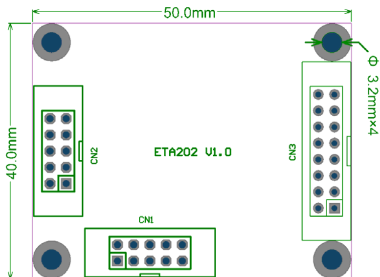
图 1: ETA202 布局图
